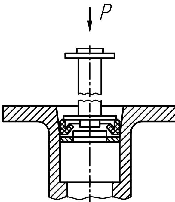
Приспособление для запрессовки манжет
